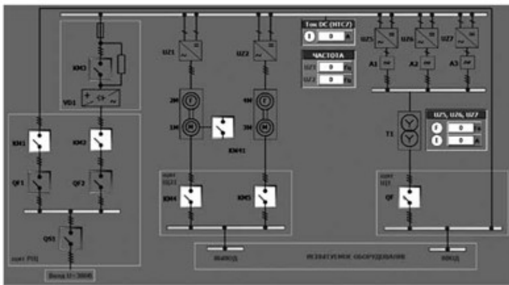
Рис. 5. Однолинейная схема стенда
